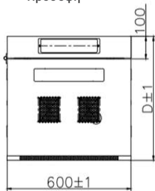
Πρόσοψη
