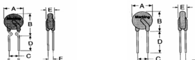
FRX 005-60F ~ FRX 090-60F Lead Size : 24AWG Φ 0.51 mm Diameter
